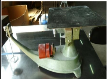
〔不等比手動はかり〕
